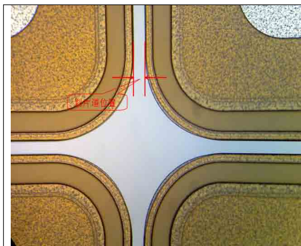
*划片道示意图
