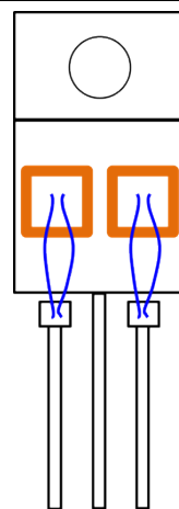
☆封装示意图 (推荐)
