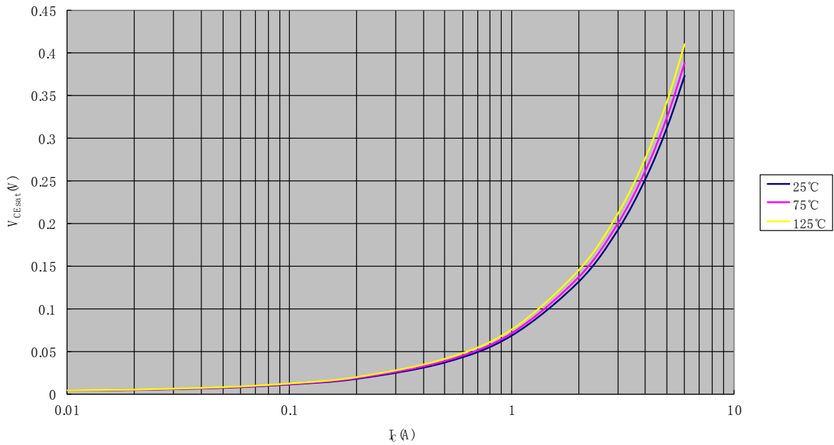
V_{CEsat} - I_C
