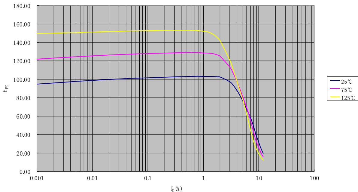
h_{FE}-I_C
