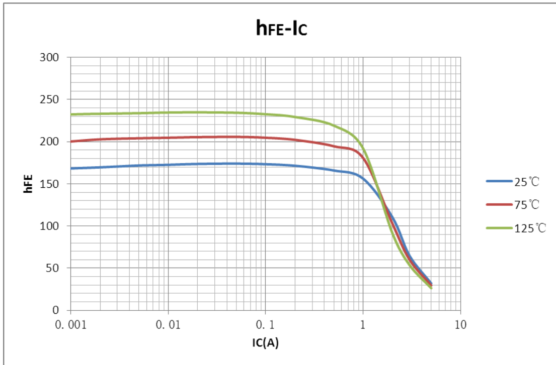
图一 h_{FE} - I_C 高温对比曲线
