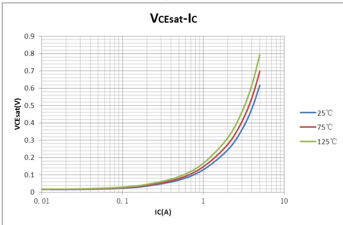
图二 V_{CEsat} - I_C 高温对比曲线
