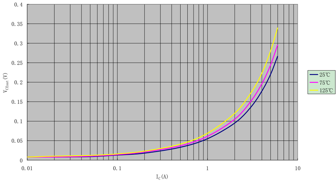
V_{CEsat}-I_C
