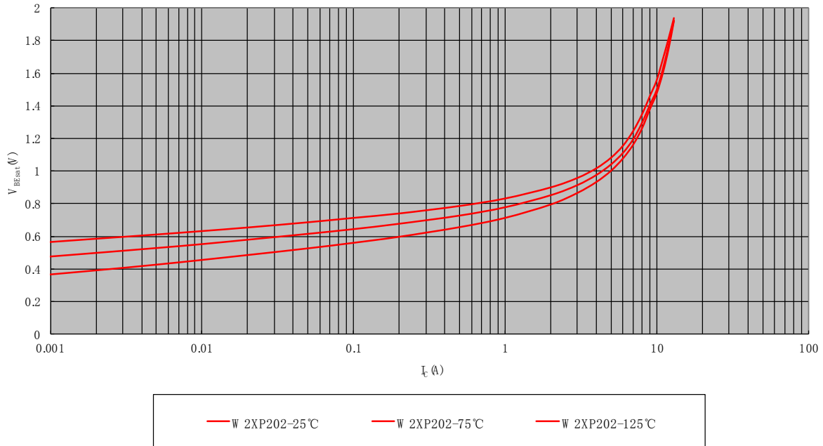
V_{BEsat}-I_C
