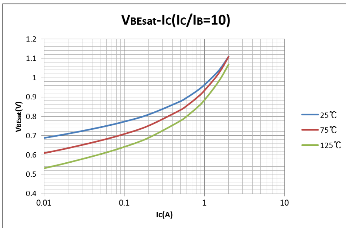
图三 V_{BEsat}-I_c 高温对比曲线
