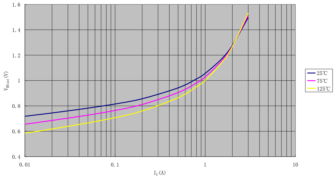
V_{BEsat}-I_C
