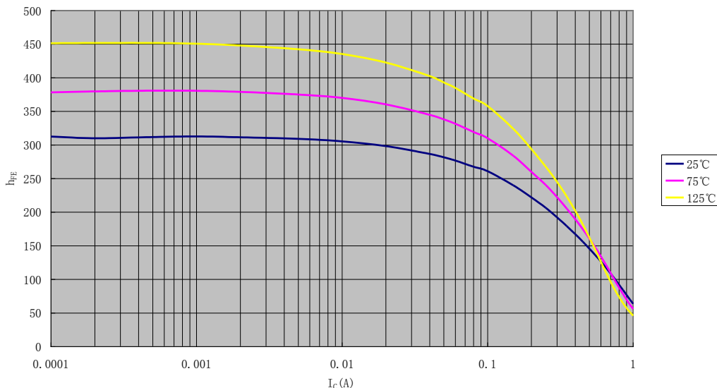
h_{FE}-I_C
