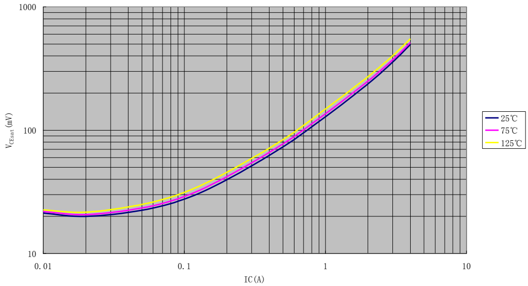
V_{CEsat}-I_C(I_C/I_B=8)
