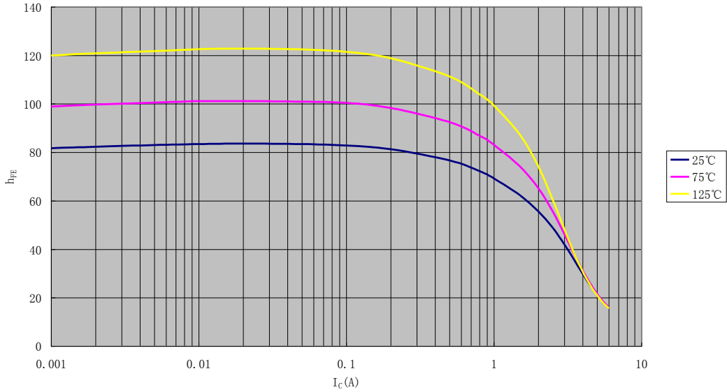
h_{FE}-I_C
