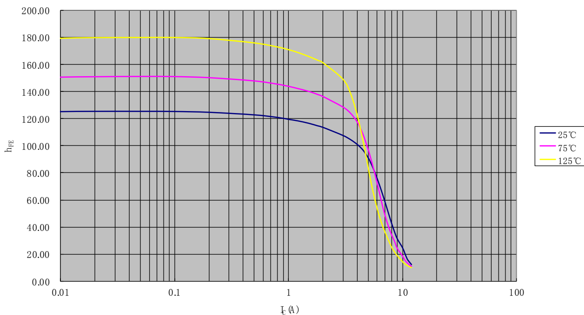
h_{FE} - I_C
